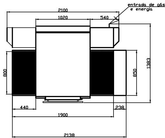
DIMENSIONAL FORNO JJ 80-103 ESTE EQUIPAMENTO PODERA SER SOBREPOSTO EM ATÉ 2 UNIDADES
