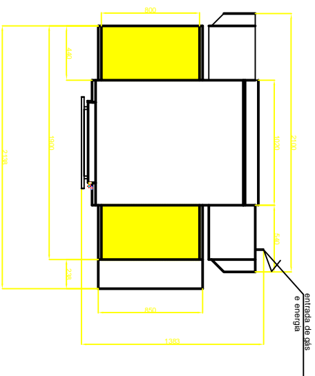
DIMENSIONAL FORNO JJA-03 ESTE EQUIPAMENTO PODERA SER SOBREPOSTO EM ATE 2 UNIDADES
