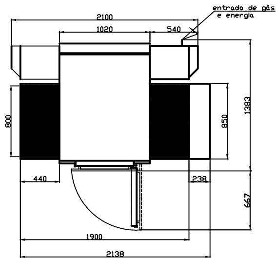
DIMENSIONAL FORNO JJ 80-103 ESTE EQUIPAMENTO PODERA SER SOBREPOSTO EM ATÉ 2 UNIDADES
