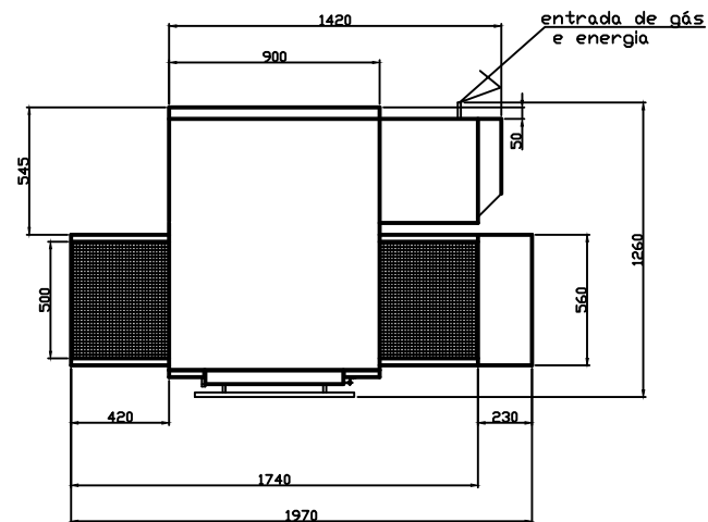
DIMENSIONAL FORNO 50-94 ESTE EQUIPAMENTO PODERA SER SOBREPOSTO EM ATÉ 2 UNIDADES
