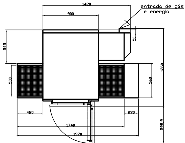
DIMENSIONAL FORNO 50-94 ESTE EQUIPAMENTO PODERA SER SOBREPOSTO EM ATÉ 2 UNIDADES
