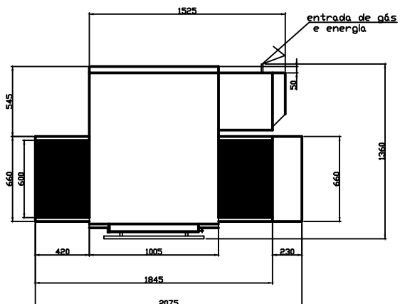
DIMENSIONAL FORNO 60-100 ESTE EQUIPAMENTO PODERA SER SOBREPOSTO EM ATÉ 2 UNIDADES
