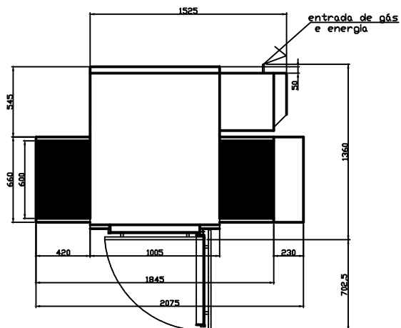
DIMENSIONAL FORNO 60-100 ESTE EQUIPAMENTO PODERA SER SOBREPOSTO EM ATÉ 2 UNIDADES
