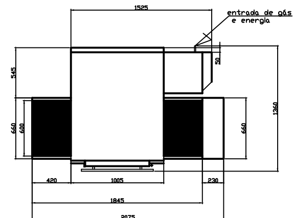
DIMENSIONAL FORNO 60-100 ESTE EQUIPAMENTO PODERA SER SOBREPOSTO EM ATÉ 3 UNIDADES
