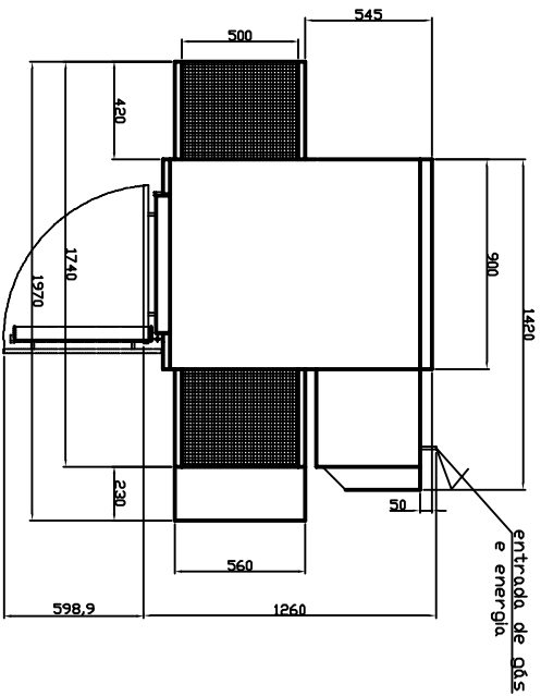
DIMENSIONAL FORNO 50-94 ESTE EQUIPAMENTO PODERA SER SOBREPOSTO EM ATE 2 UNIDADES
