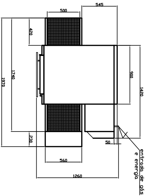
DIMENSIONAL FORNO 50-94 ESTE EQUIPAMENTO PODERA SER SOBREPOSTO EM ATE 2 UNIDADES
