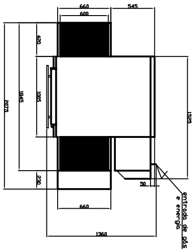
DIMENSIONAL, FORNO 60-100 ESTE EQUIPAMENTO PODERIA SER SOBREPOSTO EM ATÉ 3 UNIDADES
