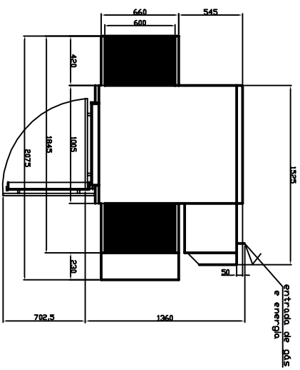
DIMENSIONAL, FORNO 60-100 ESTE EQUIPAMENTO PODERIA SER SOBREPOSTO EM ATÉ 2 UNIDADES
