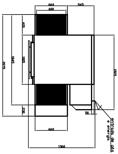
DIMENSIONAL, FORNO 60-100 ESTE EQUIPAMENTO PODERIA SER SOBREPOSTO EM ATÉ 2 UNIDADES
